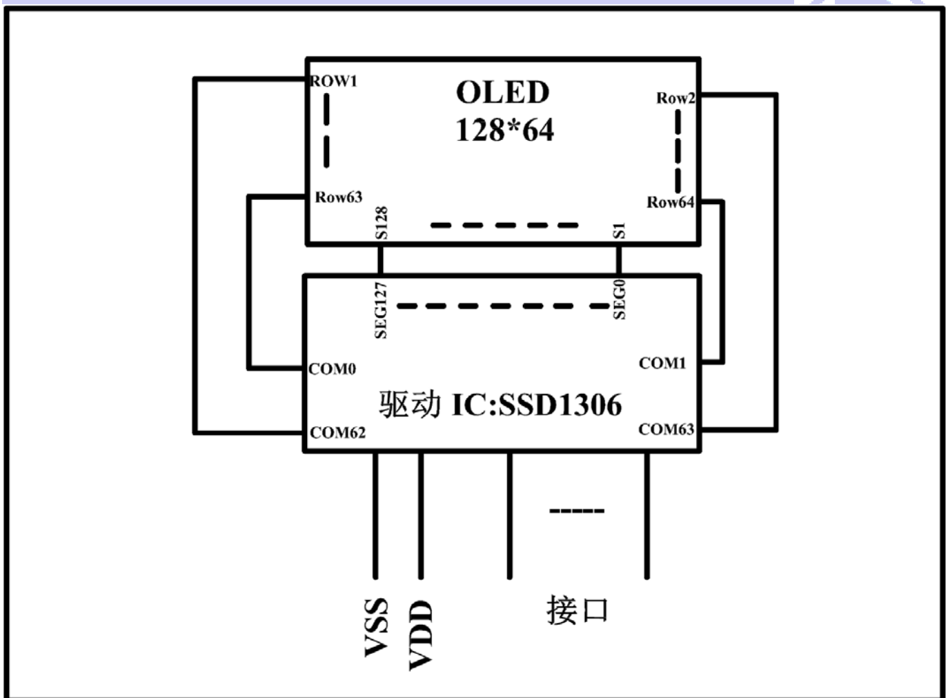
图 2. JLX12864OLED-096-PN-12C
