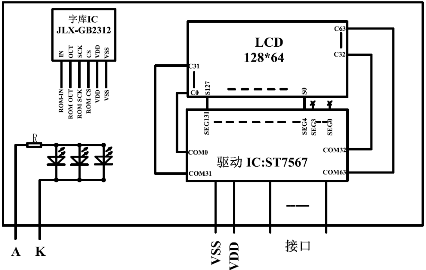
图 2: JLX12864G-13605 电路框图
